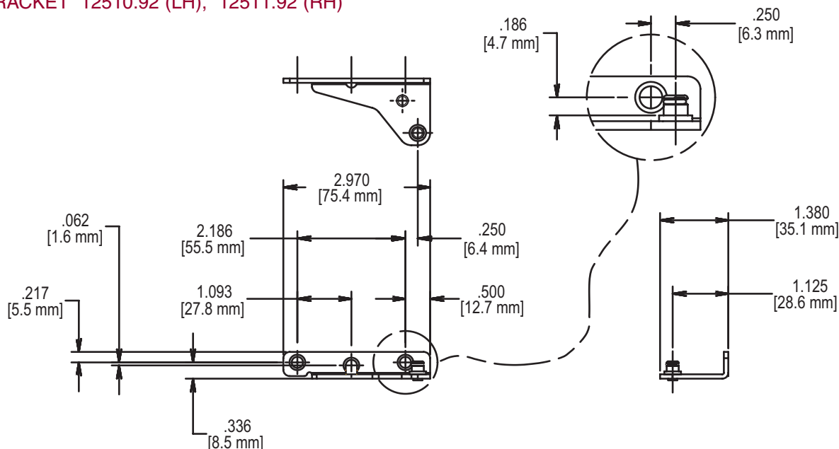
FIG. 5 BRACKET 12510.92 (LH), 12511.92 (RH)
