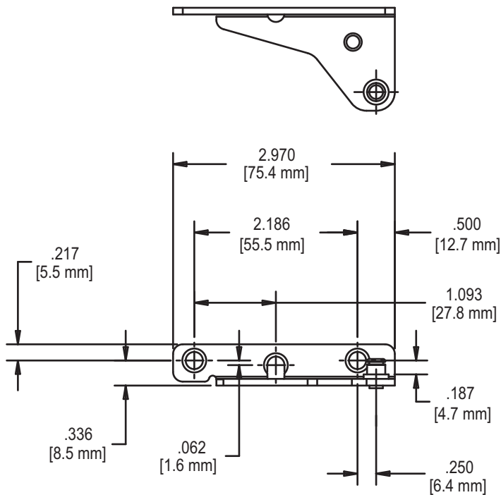
FIG. 4 STUD BRACKETS 12512.XX, 12513.XX
