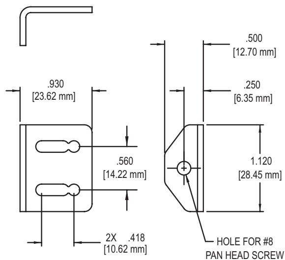
FIG. 7 STABILIZING TAB 12789
