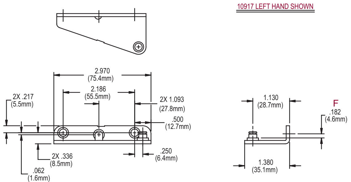
FIG. 8 STUD BRACKETS 10917.XX, 10918.XX
